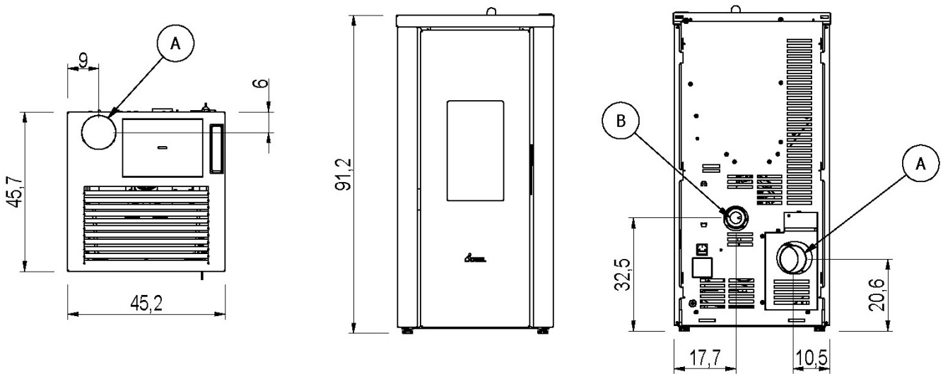
Fig. 14 - Dimensioni generali:VERA 7.0 UP
