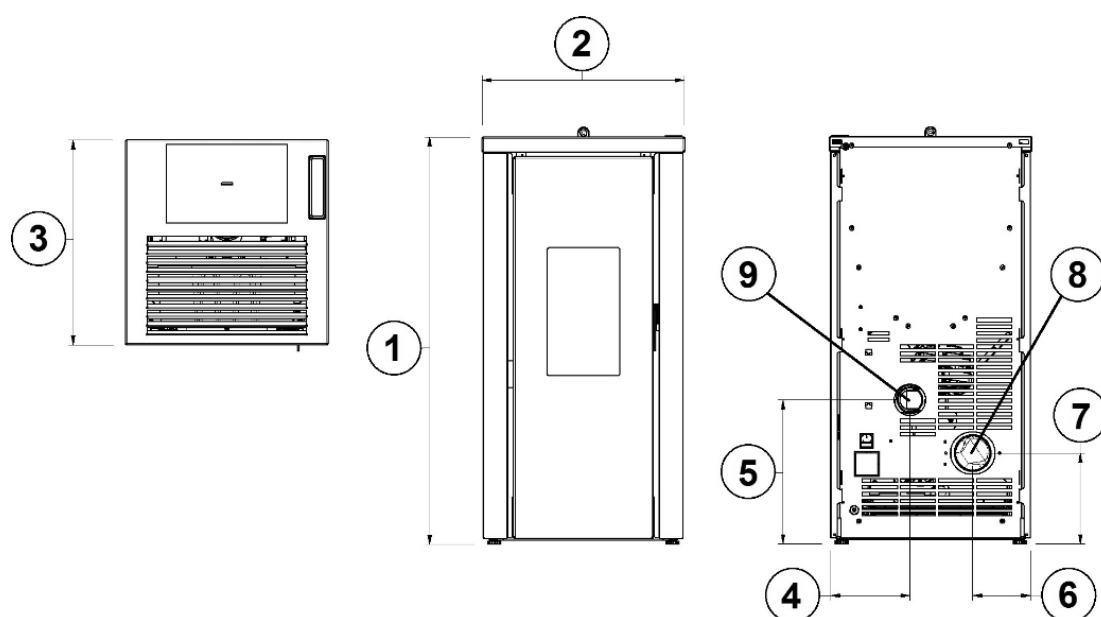
Fig. 12 - Dimensioni generali: VERA 7 - VERA 7.0
