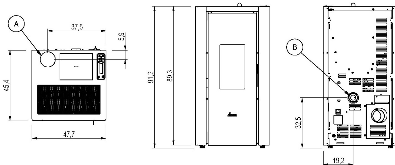
Fig. 15 - Dimensioni generali:CRISTAL7.0 UP
