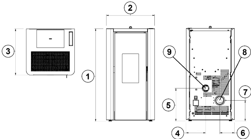
Fig. 13 - Dimensioni generali:INDIGO EVO - INDIGO EVO 7
