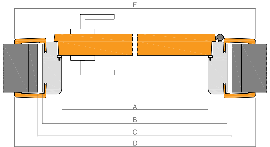
SEZIONE ORIZZONTALE
