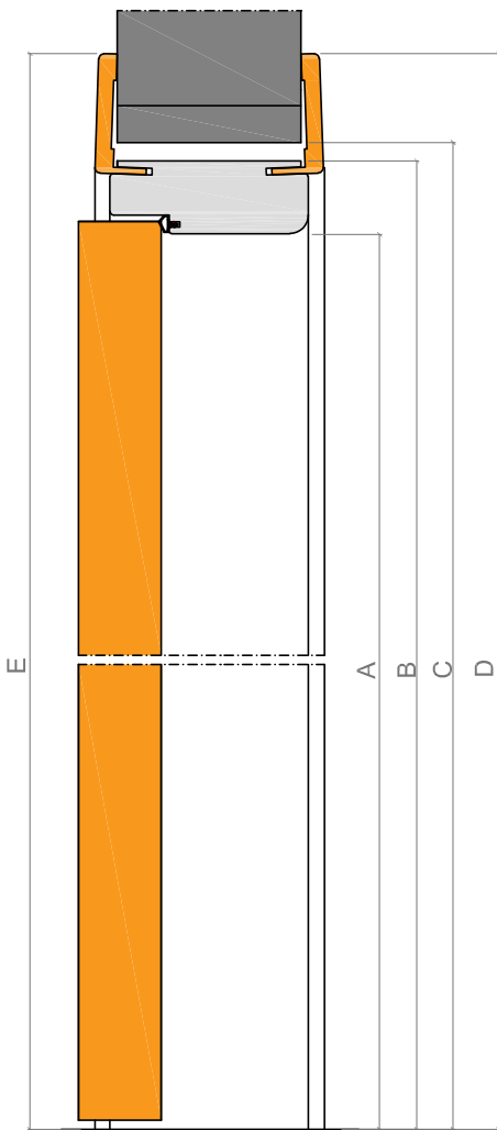
SEZIONE VERTICALE
