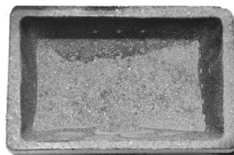
Fig. 34 - Esempio di braciere sporco
