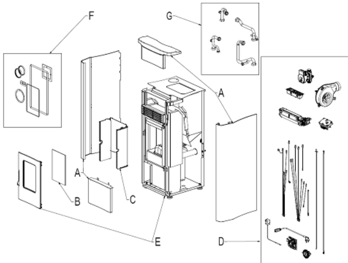
Fig. 1 - Esploso
